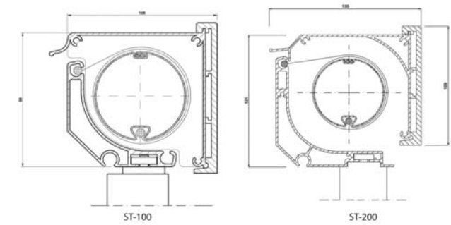
Tekening van de gesloten cassettevorm
